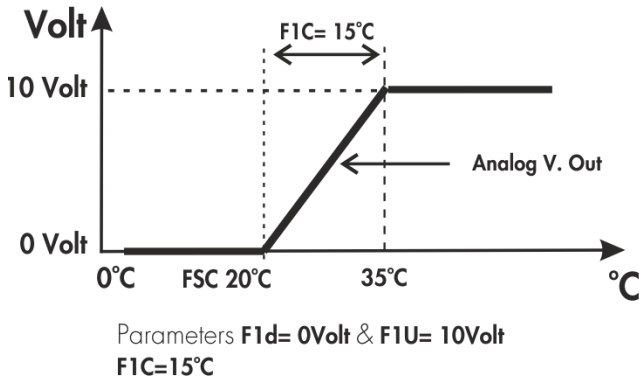
ΣΧΗΜΑ 6A FAN 1 ΣΤΗΝ ΨΥΞΗ
