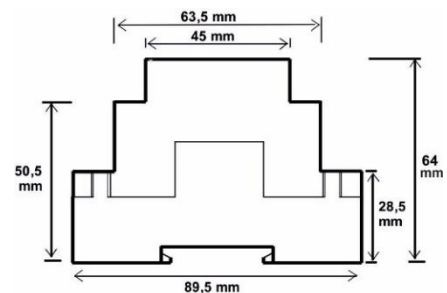
ΣΧΗΜΑ 3 ΔΙΑΣΤΑΣΕΙΣ
