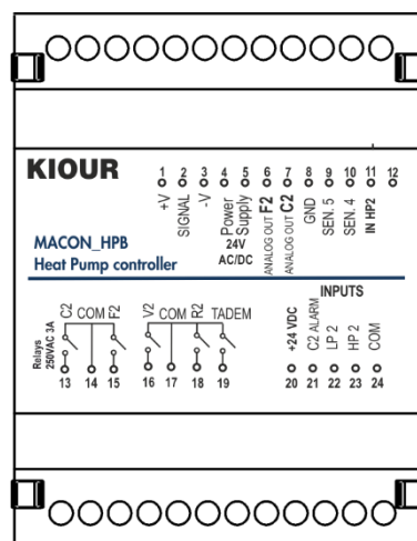
ΣΧΗΜΑ 2 MACON_HPB
