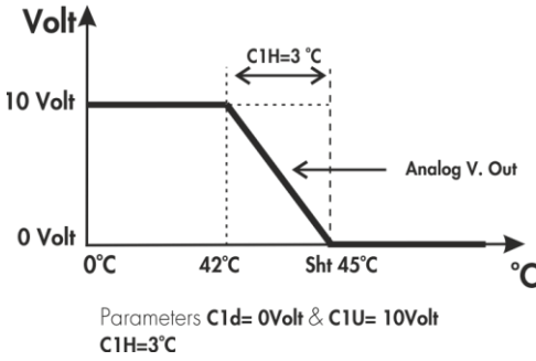
ΣΧΗΜΑ 5B ΣΥΜΠΙΕΣΤΗΣ C1 ΣΤΗΝ ΘΕΡΜΑΝΣΗ
