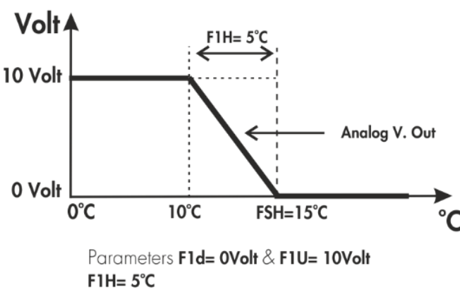
ΣΧΗΜΑ 6B FAN 1 ΣΤΗΝ ΘΕΡΜΑΝΣΗ
