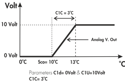
ΣΧΗΜΑ 5A ΣΥΜΠΙΕΣΤΗΣ C1 ΣΤΗΝ ΨΥΞΗ
