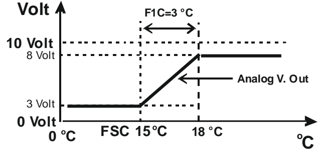
Parameters F1d=3.0 Volt & F1U=8.0 Volt F1C=3°C
