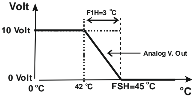
Parameters F1d=0 Volt & F1U=10 Volt F1H=3°C
