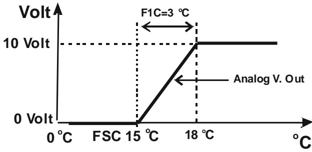
Parameters F1d=0 Volt & F1U=10 Volt F1C=3°C
