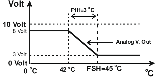
Parameters F1d=3.0 Volt & F1U=8.0 Volt F1H=3°C
